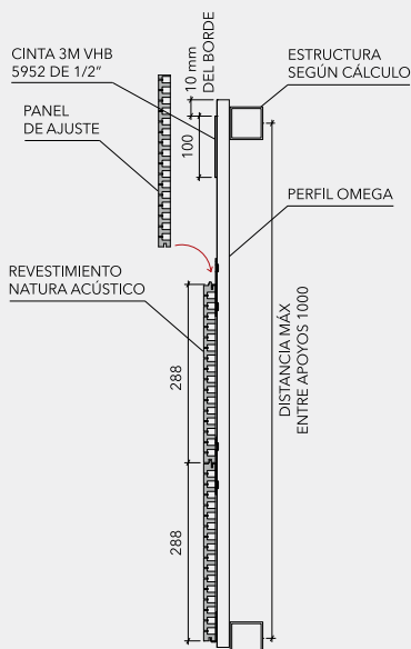
CORTE A-A
