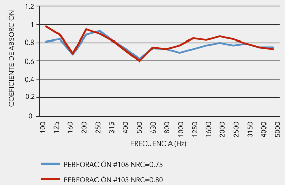
CIELO TILE GRÁFICO COEFICIENTE ABSORCIÓN ACÚSTICA V/S FRECUENCIA
